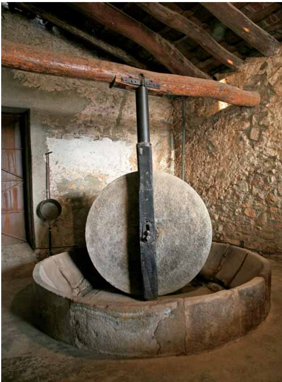
El trull per a fer oli de can Mataporcs.
